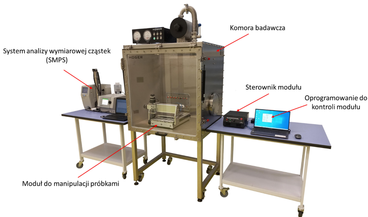
Rysunek 1. Widok stanowiska do badania emisji nanoobjektów z materiałów z materiałów użytkowych pokrytych warstwami funkcjonalnymi
