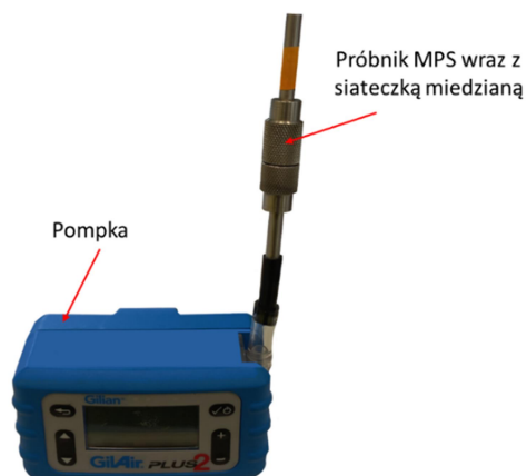
Rysunek 4. Widok próbnika MPS wraz z pompką indywidualną
