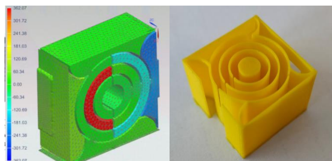
Rys. 3. Wyniki badania numerycznego rezonansów własnych układu wielopięścieniowego oraz widok komórki metamateriału drukowany techniką 3D
