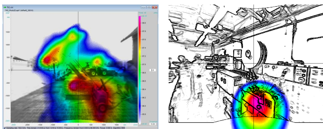
Rys. 5. Wizualizacje hałasu przy przecinaniu pakietu desek piłą mobilną (po lewej) oraz hałasu drukarki fleksograficznej (po prawej) wykonane z wykorzystaniem kamer akustycznych.
