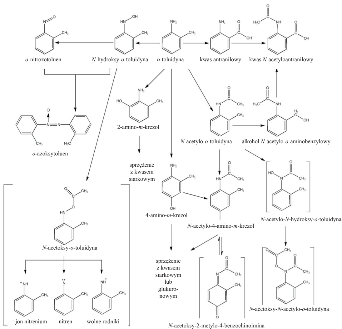
Rys. 2. Schemat przemian metabolicznych 2-toliloaminy (NTP 2014)
